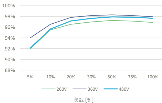
效率曲线
