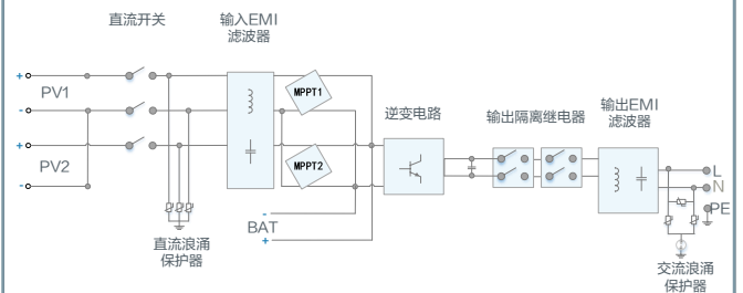
电路框图
