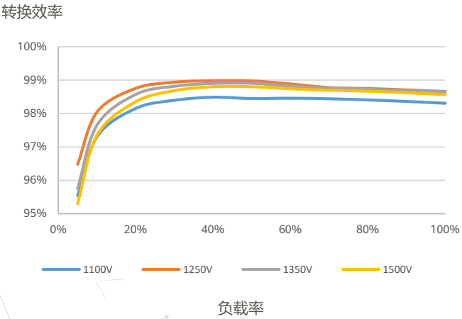
效率曲线
