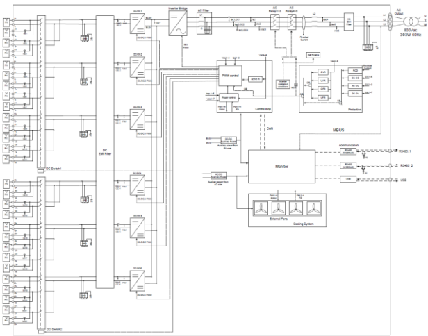
电路框图
