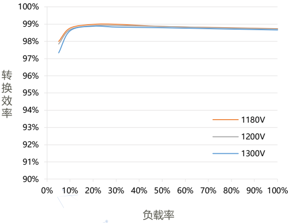
效率曲线
