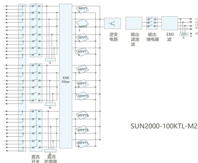
电路框图
