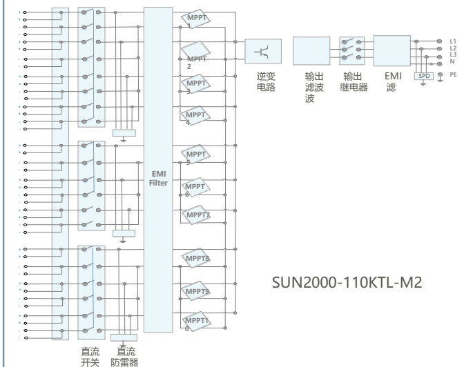
电路框图
