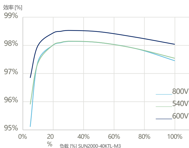
效率曲线
