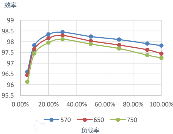
效率曲线
