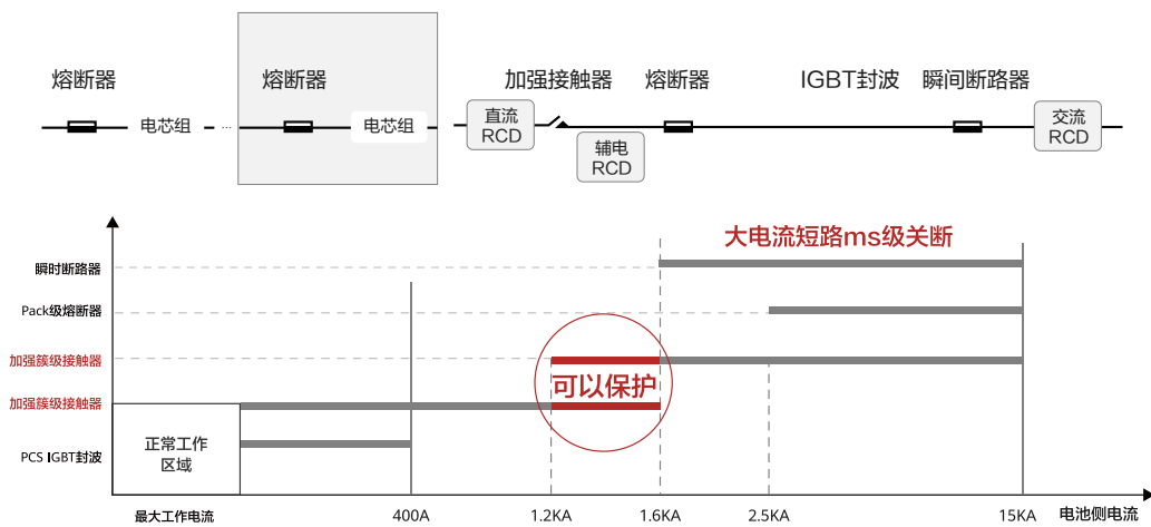
图27. 系统级五级全保护原理图
