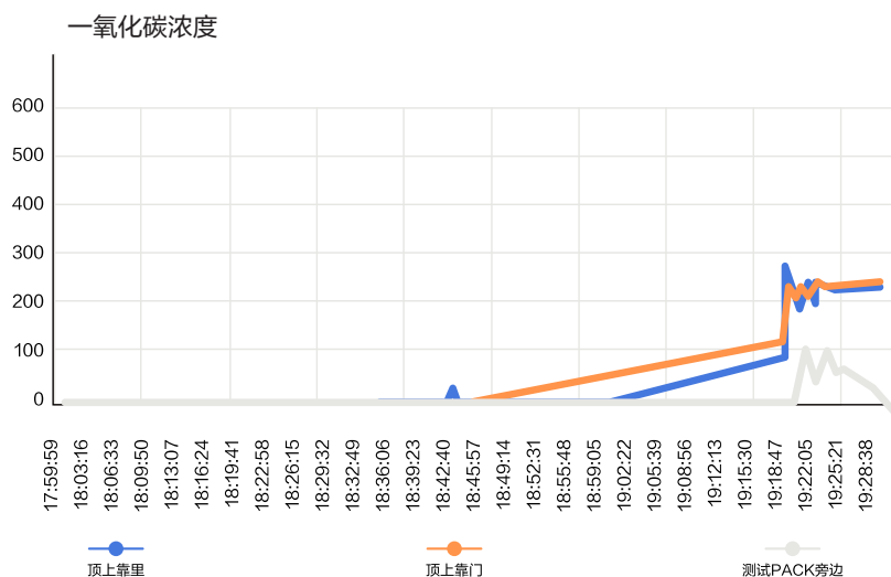
图35. 定向排烟效果测试及柜内可燃气体浓度检测
