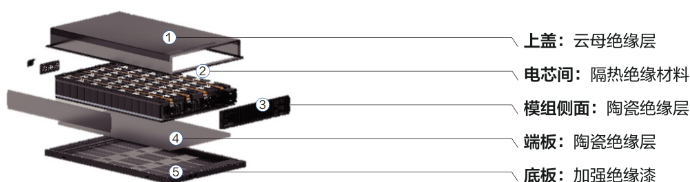
图25. 电池包六面绝缘设计
