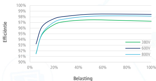
Efficiëntiecurve
