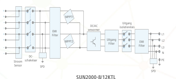
Schakelschema
