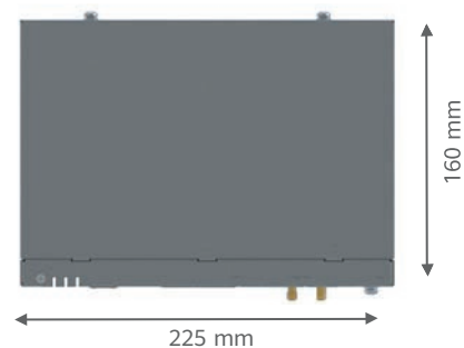
3000A00(LITE版)
