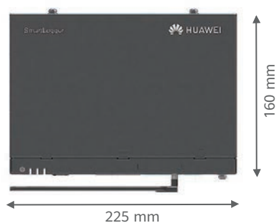
SmartLogger 3000A
