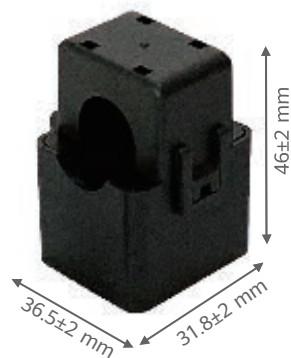
SmartPS2000-100-A
