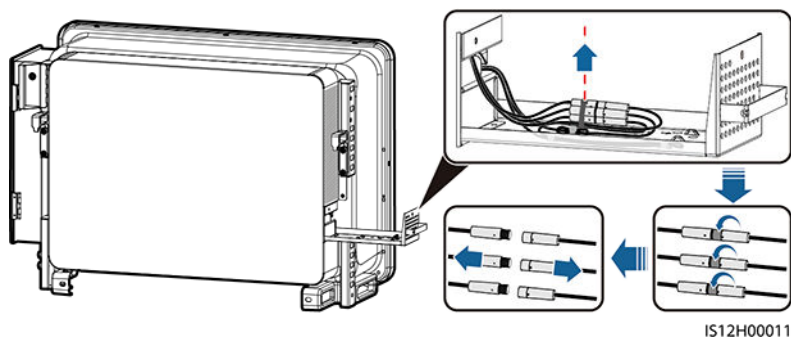
Εικόνα 8-5 Καλώδια αποσύνδεσης
