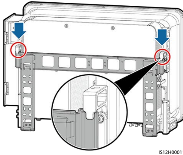
Εικόνα 4-18 Τοποθέτηση του ηλιακού αντιστροφέα
