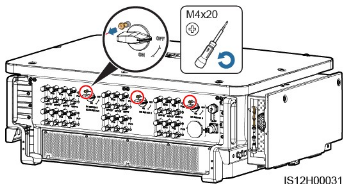
Εικόνα 6-1 Αφαιρέστε τις βίδες
