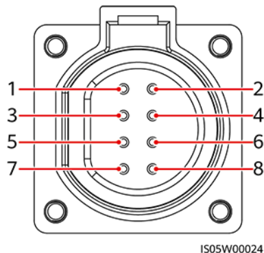
Εικόνα 5-25 Θύρα επικοινωνιών
