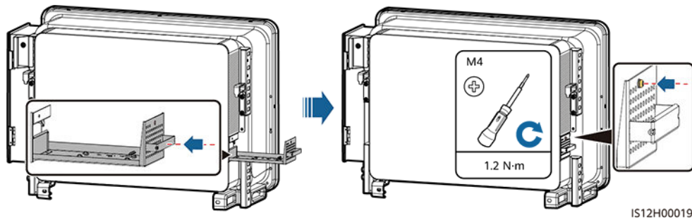
Εικόνα 8-17 Επανατοποθέτηση του δίσκου του ανεμιστήρα
