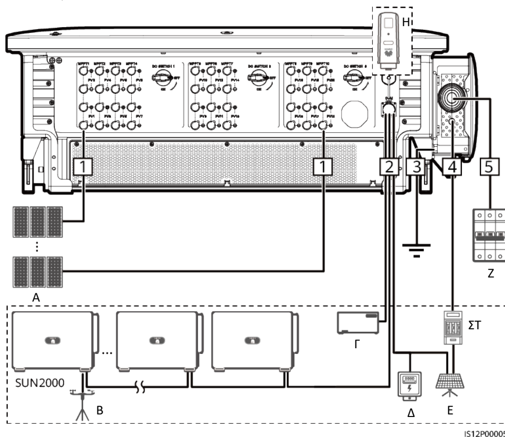
Εικόνα 5-5 Συνδέσεις καλωδίων (διαμορφώστε τα εξαρτήματα στο πλαίσιο με κουκκίδες όπως απαιτείται)
