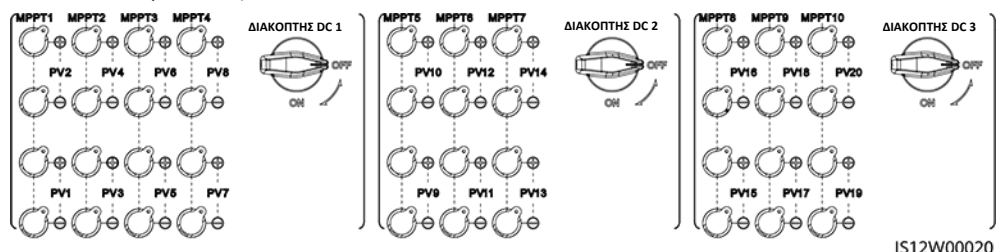
Εικόνα 5-20 Ακροδέκτες DC
