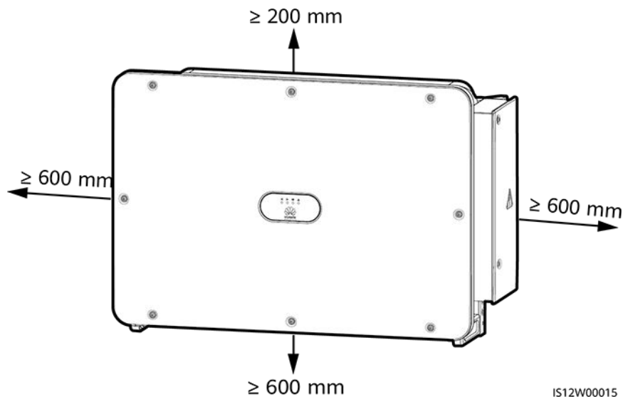
Εικόνα 4-4 Διαστάσεις εγκατάστασης
