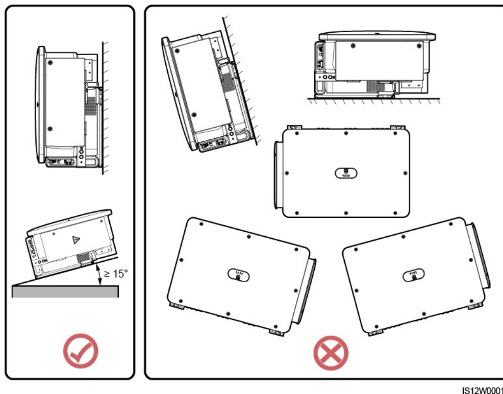
Εικόνα 4-3 Γωνία
