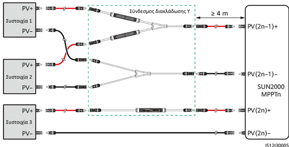
Εικόνα 5-23 Σύνδεση των συνδέσμων διακλάδωσης Y στον ηλιακό αντιστροφέα
