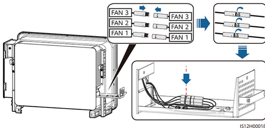
Εικόνα 8-16 Επανασύνδεση και πρόσδεση των καλωδίων
