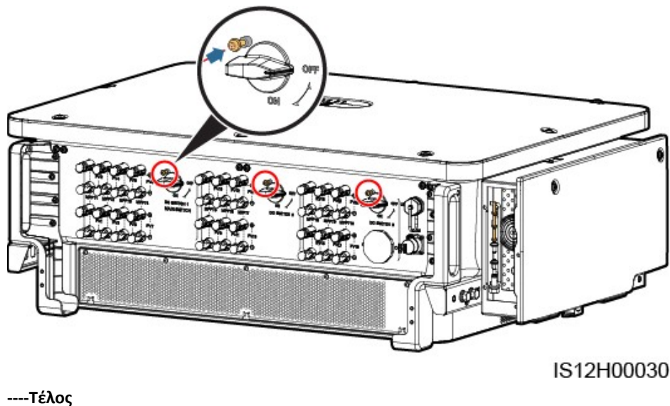
Εικόνα 8-1 Τοποθετήστε τις βίδες για το κλείδωμα των διακοπών DC
