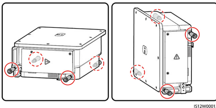
Εικόνα 4-12 Θέσεις για την τοποθέτηση των λαβών
