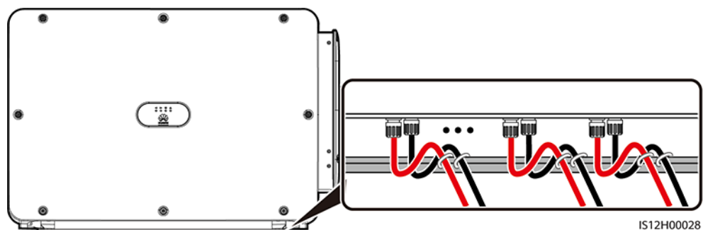
Σχήμα A-6 Πρόσδεση συνδέσμων διακλάδωσης Υ
