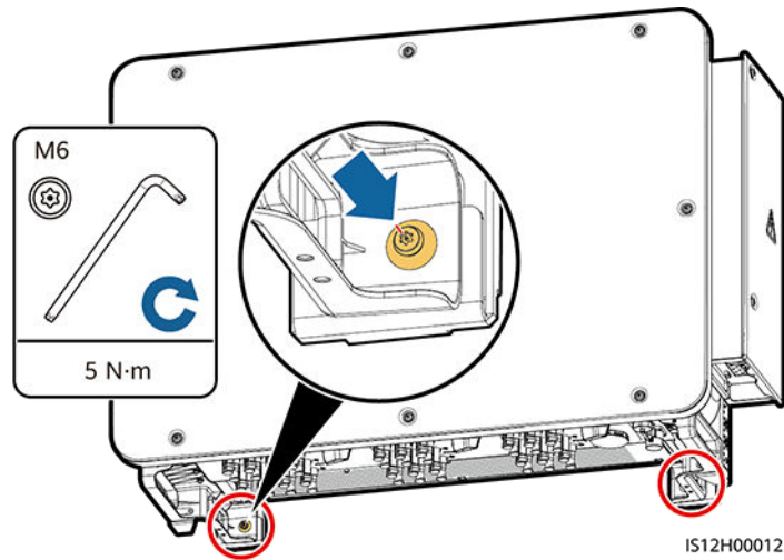
Εικόνα 4-19 Σύσφιγξη των βιδών Torx ασφαλείας
