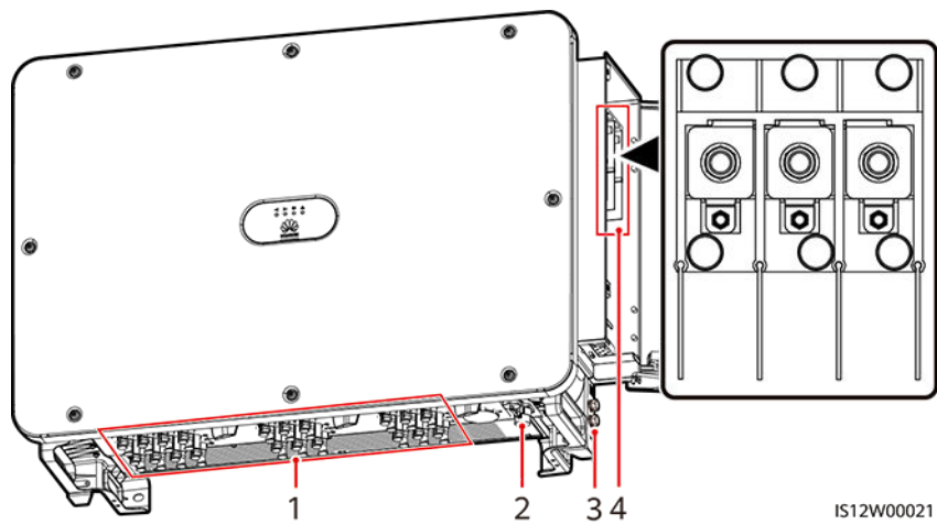
Εικόνα 2-8 Θύρα καλωδίωσης μοντέλου 3 ακίδων (SUN2000-125KTL-M0)
