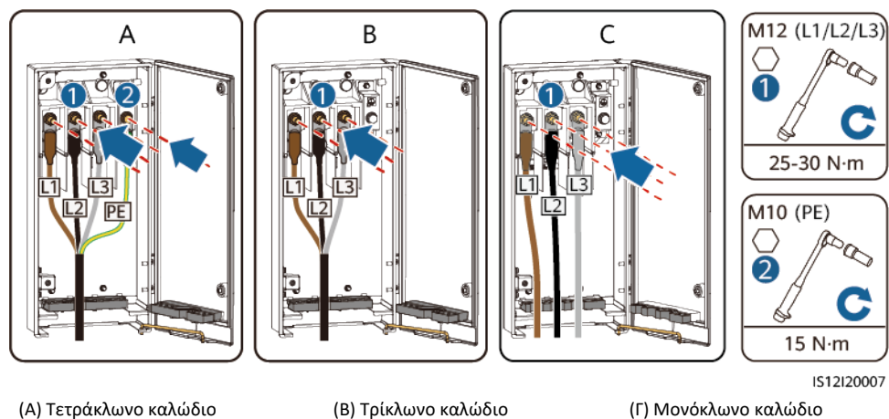
Εικόνα 5-18 Συνδέσεις καλωδίων μοντέλου 3 ακίδων (125KTL)
