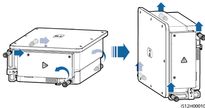
Εικόνα 4-16 Ανύψωση του ηλιακού αντιστροφέα και διατήρηση του σε όρθια θέση
