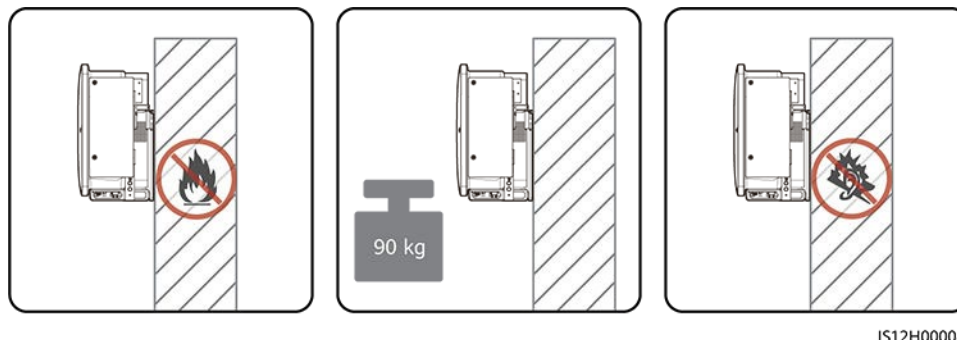
Εικόνα 4-2 Δομή τοποθέτησης
