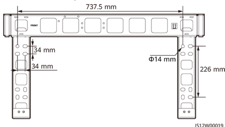
Εικόνα 4-9 Διαστάσεις οπών
