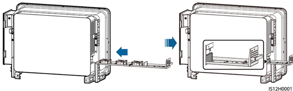
Εικόνα 8-15 Ωθήστε τον δίσκο του ανεμιστήρα προς τα μέσα
