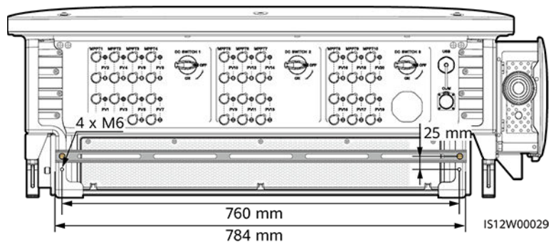
Εικόνα A-4 Συνιστώμενες διαστάσεις
