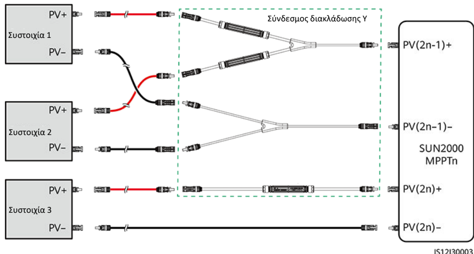
Εικόνα 5-23 Σύνδεση των συνδέσμων διακλάδωσης Y στον ηλιακό αντιστροφέα
