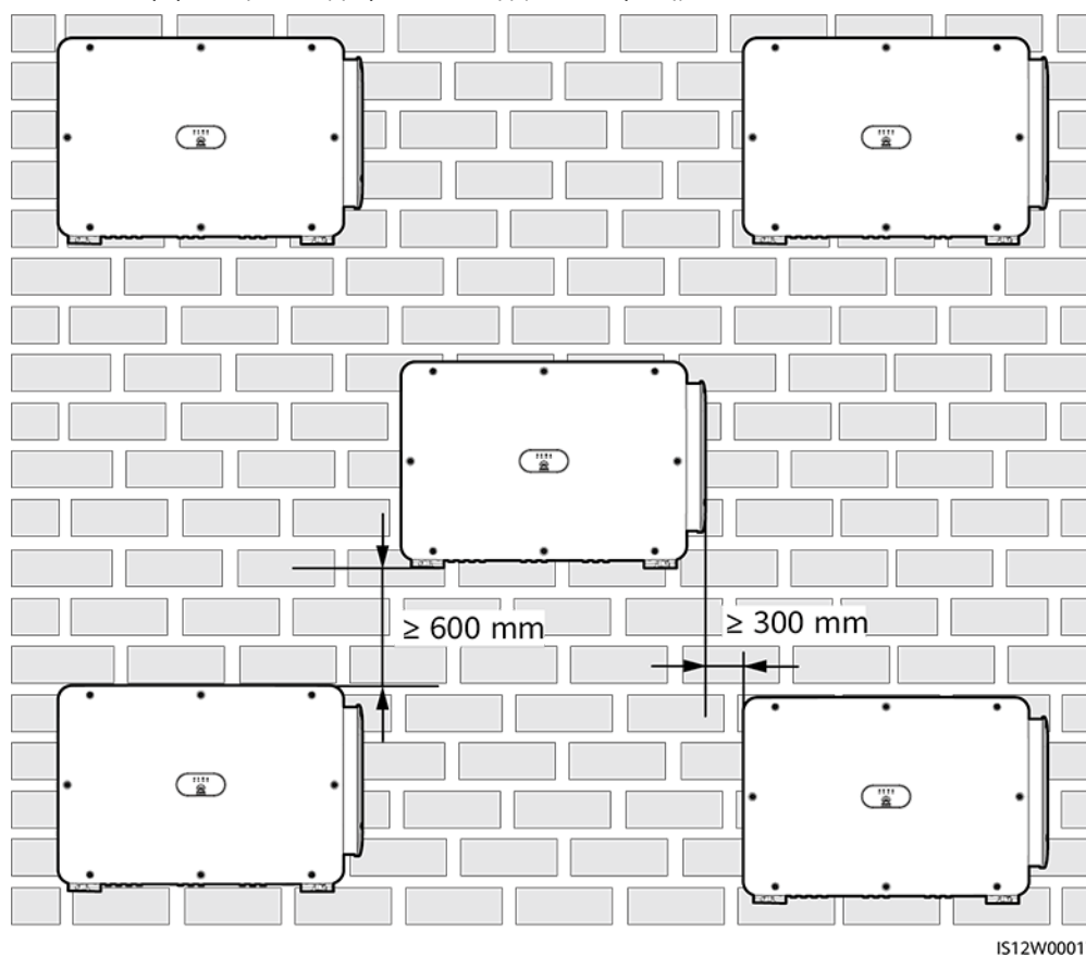
Εικόνα 4-6 Τριγωνική διάταξη εγκατάστασης (συνιστώμενη)
