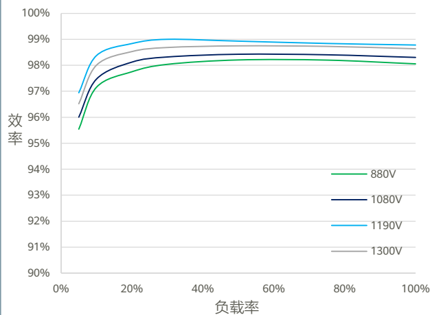
效率曲线
