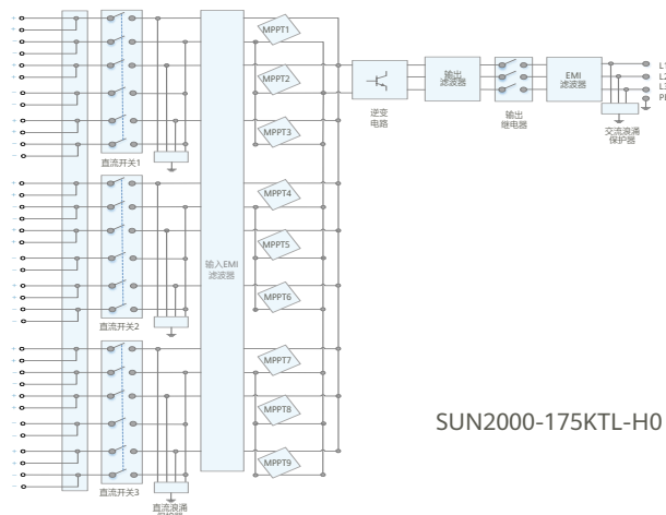
电路框图
