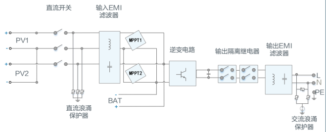
电路框图
