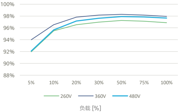
效率曲线
